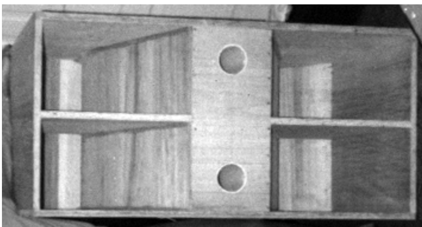
Foto 4 - W-Horn JBL divulgada no Brasil e sintonizada por CCDB
