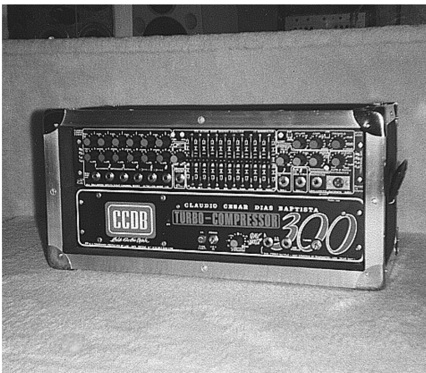
Foto 25 - TURBO-COMPRESSOR 300 CCDB
