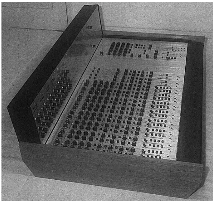
Foto 30 - Mesa modular de gravação CCDB Série III
