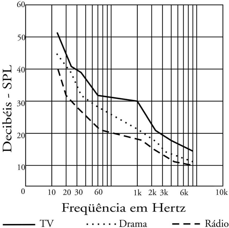
Figura 1 - Ruído de fundo permissível em estúdios
