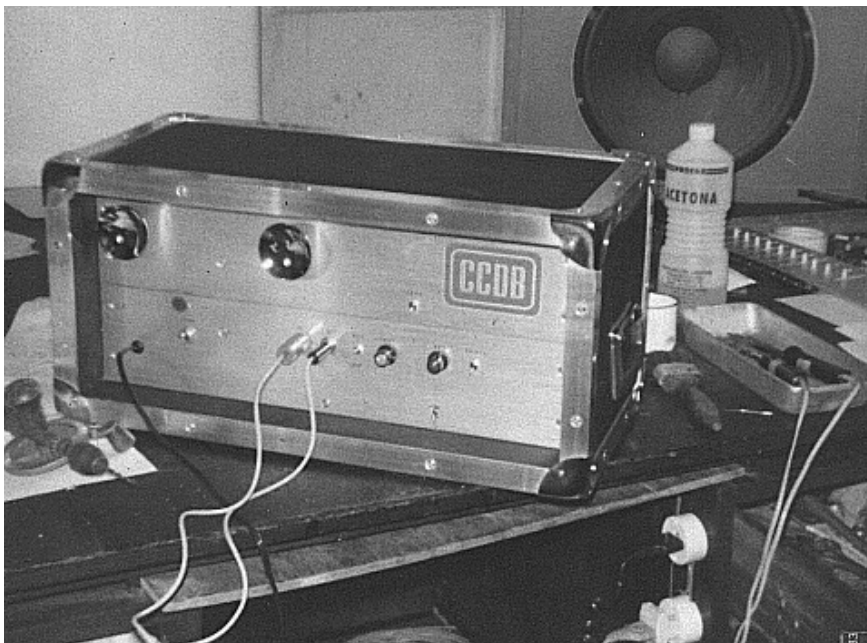
Foto 16 - Câmara de reverberação CCDB, com molas
